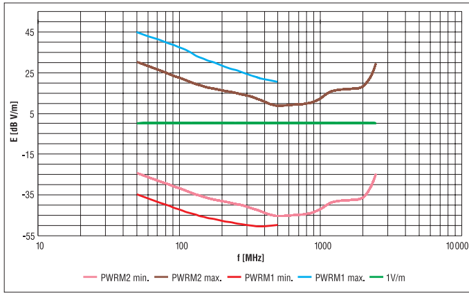
Bild 6: Nutzbare Meßbereichsgrenzen BMA1 mit PWRM1 und PWRM2
