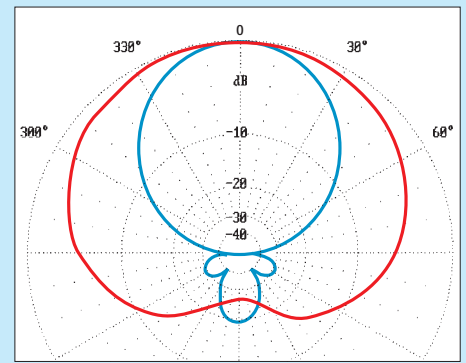
Bild 3: Richtdiagramm der HB9CV-Antenne (rot) im Vergleich zur 3-Element-Yagi, bezogen auf Vertikalpolarisation. Plots: DK7ZB
