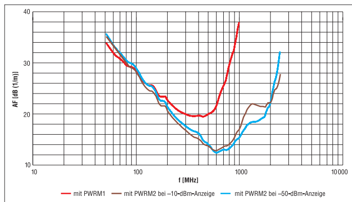
Bild 5: Über-alles-Antennenfaktoren für die Kombinationen BMA1 mit PWRM1 bzw. PWRM2 (BMA1 über BNC-Kupplung mit PWRM1 bzw. PWRM2 direkt verbunden)
