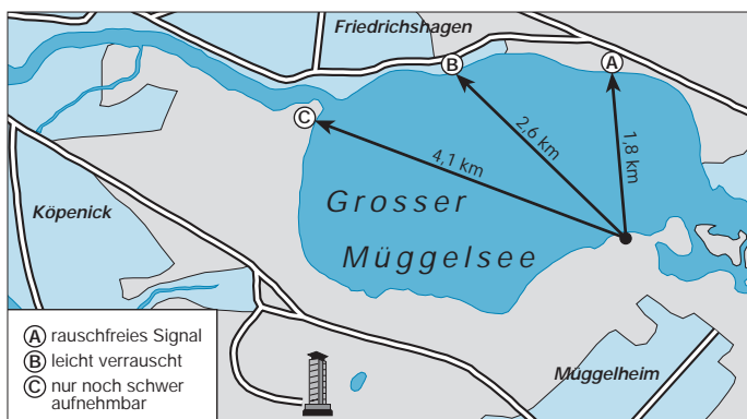
Bild 5: Die Reichweite des VX-246 wurde auch anhand dreier verschieden weit entfernter Zielkoordinaten quer über den Berliner Müggelsee getestet ...
