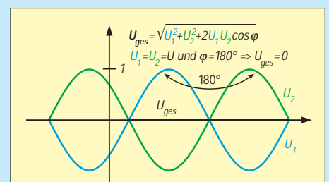
Bild 4: Auslöschung nach hinten durch Überlagerung 180^\circ verschobener Wellenzüge
