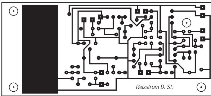
Bild 2: Platinenlayout
