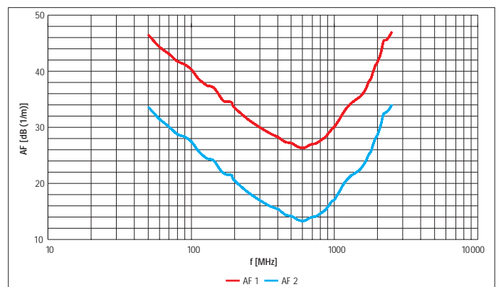
Bild 2: Antennenfaktoren für BMA1 in Kombination mit frequenzlinearem dBµV- bzw. dBm-Pegelmessgerät
