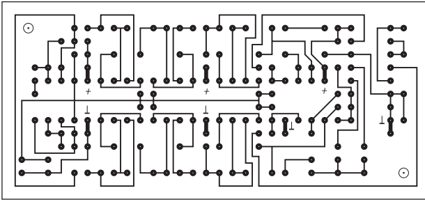
Bild 12: Ein mögliches Layout für den Allpaß-Block
