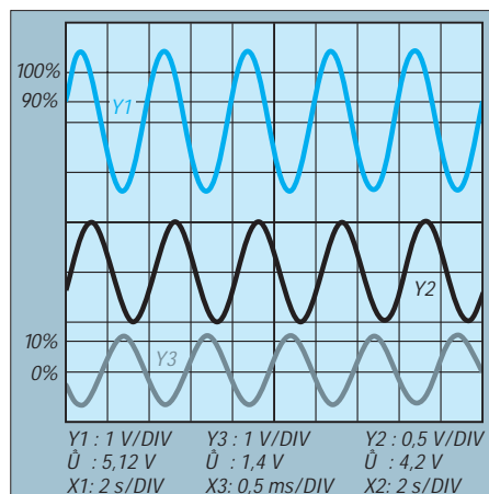
Bild 4: Oszillogramme zu Bild 2. Y1: Ausgangsspannung an A; Y2: Spannungsverlauf am Ausgang von N2.1; Y3: Spannungsverlauf am Ausgang von N2.2
