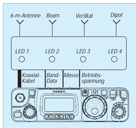
Bild 4: Zusammenschaltungsvariante
