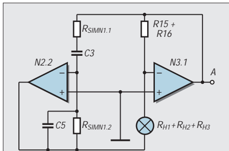
Bild 1: Funktionsprinzip des hier beschriebenen Generators mit Wien-Robinson-Brücke
