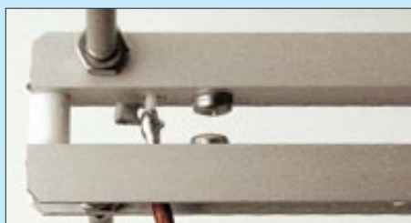
Bild 6: Parallel zur Speiseleitung liegt ein Kondensator von 5,6 pF, siehe auch Bild 12.
