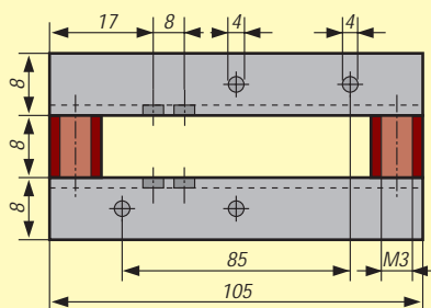
Bild 11: Ansicht von der Seite auf beide Boomstreben, nicht maßstäblich
