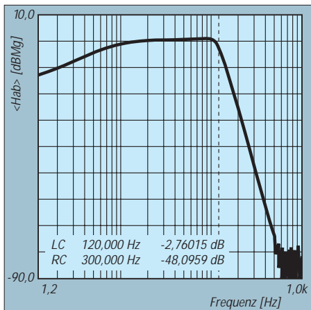
Bild 5: Frequenzgangkennlinie, aufgenommen mittels eines R9211B-FFT-Servoanalyzers
