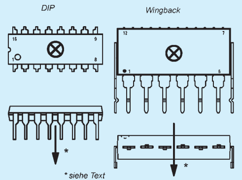
Bild 4: Die Gehäuse der MMA-Serie unterscheiden sich durch die Meßrichtungen.
