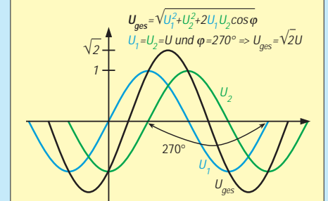
Bild 5: Verstärkung nach vorn infolge 270^\circ Phasenverschiebung
