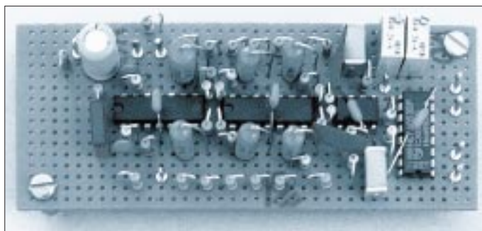
Bild 11: Musteraufbau des Allpaß-Blocks
