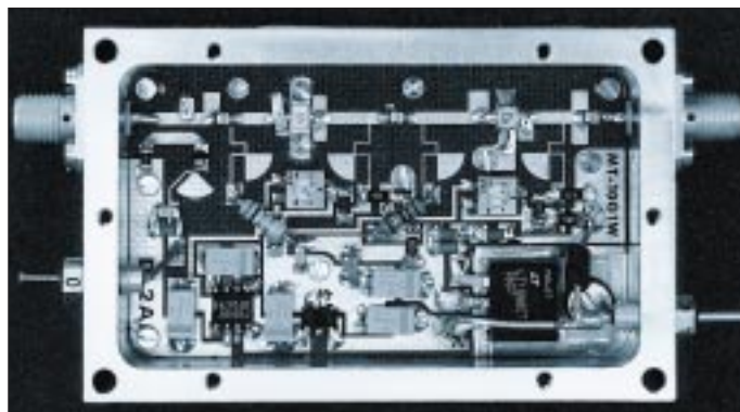
Fertig aufgebautes 10-GHz-Endstufenmodul von DL2AM
