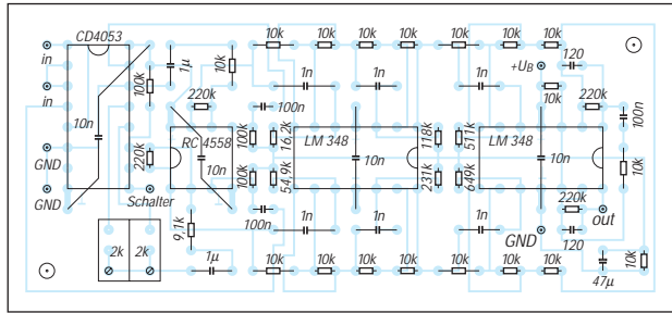
Bild 13: Bestückungsplan für Platinen- oder Lochrasterplatten-Aufbau; die auf der Leiterseite mit + bzw. ↓ gekennzeichneten Betriebs-spannungsanschlüsse sind jeweils durch Drähte auf der Leiterseite untereinander zu verbinden.
