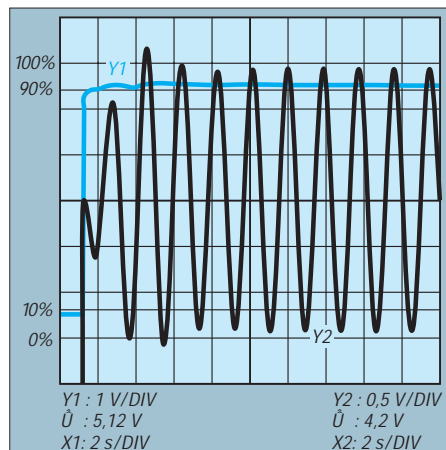
Bild 3: Oszillogramme zu Bild 2. Y1: Verlauf von U_S nach dem Einschalten; Y2: Ausgangsspannung an A
