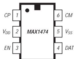
Bild 1: Pinbelegung des MAX 1474
