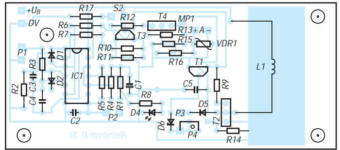
Bild 3: Bestückungsplan
