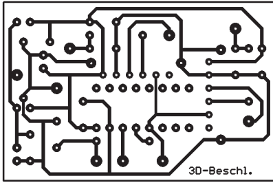
Bild 7: Bei dem minimalen Bauelemente-aufwand wäre fast keine Platine notwendig.
