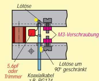
Bild 12: Einspeisung im Detail; die untere Lötöse dient auch zur Zugentlastung.
