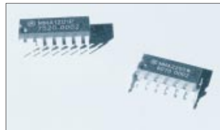
Bild 2: Die Beschleunigungssensoren von MOTOROLA gibt es im DIP und Wingback-Gehäuse.
