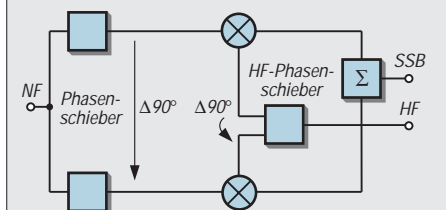
Bild 18: Für die Anwendung modifiziertes Prinzip der Modulation
