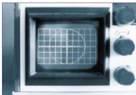
Bild 16: Makelloser Schirmbild bei 1 kHz. Das Sprachspektrum ist hier am stärksten ausgeprägt, die Schaltung darum auf diese Frequenz optimiert. Bei Frequenzänderungen gibt es leicht zu erkennende Abweichungen von der Idealform. Fotos: DL7VFS
