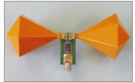
Bild 3: BMA1-Meßdipol 50 MHz bis 2,5 GHz Anschluß BNC, 50 Ω Zwangsanpassung erforderlich, Dipol-Abmessungen L × B 178 mm × 68 mm, Masse 100 g [5]
