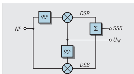
Bild 17: Prinzip der SSB-Modulation nach der Phasenmethode
