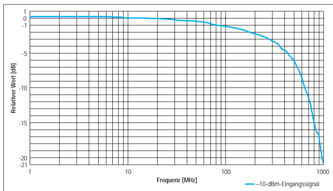
Bild 4: Typischer Anzeigefrequenzgang des PWRM1
